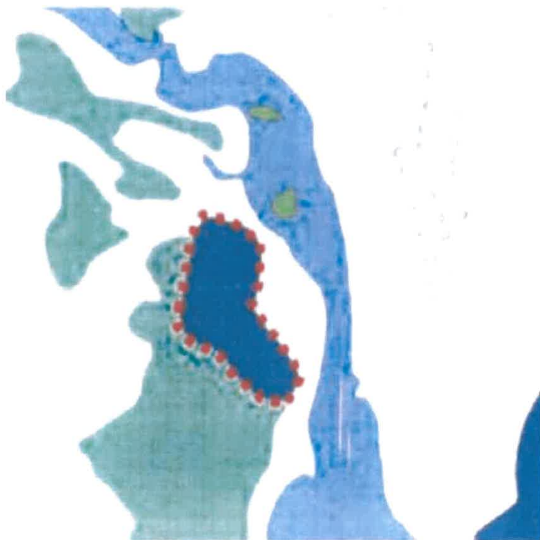
Рисунок 27 - Карта-схема места обитания Большой выпи
