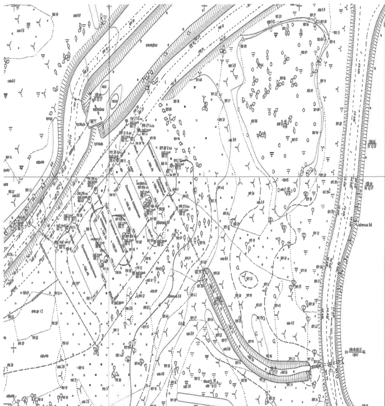
Рисунок 7 – Очистные сооружения в районе ул. Чижевских
