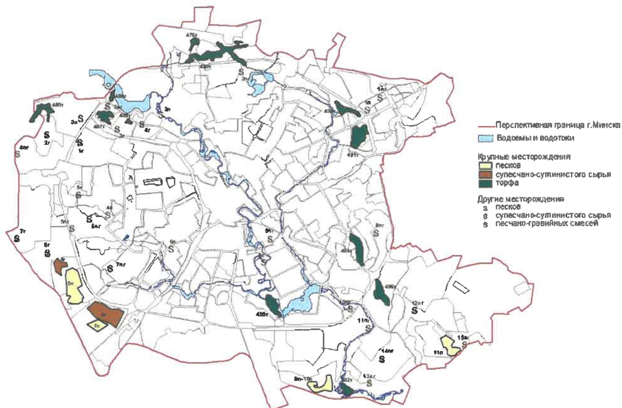
Рисунок 13 - Карта месторождений полезных ископаемых на территории г.Минска
